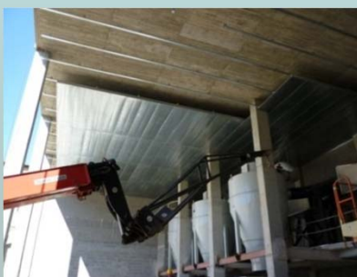
Techo con pantallas acústicas
